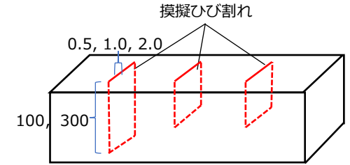
ひび割れ供試体のイメージ
