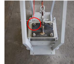
ボルトの緩み試験体例
