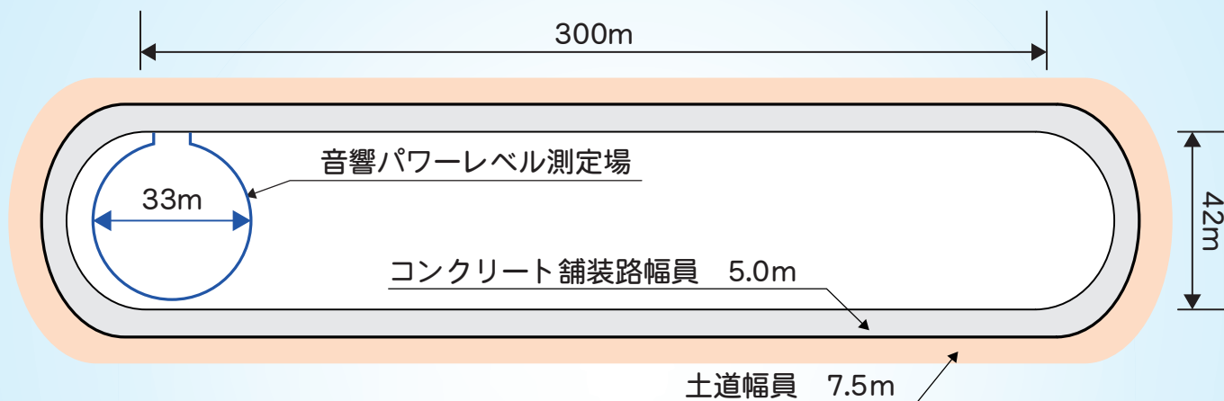
テストコース概要(1周:750m)
