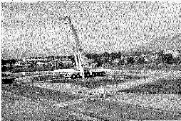
写真一七 音響パワーレベル測定状況
