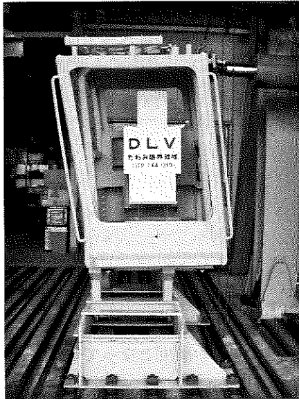
写真一六 ROPS 側方載荷試験状況
