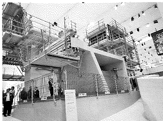
写真-19 作業床 (PERI)
