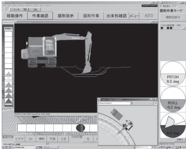
図-4 操作インターフェースの画面（例）
