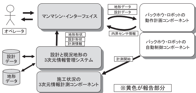
図一 バックホウ・ロボットのシステムの構成
