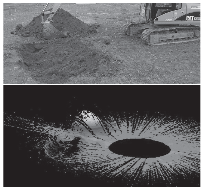
図一3 レーザスキャナによる測定結果
