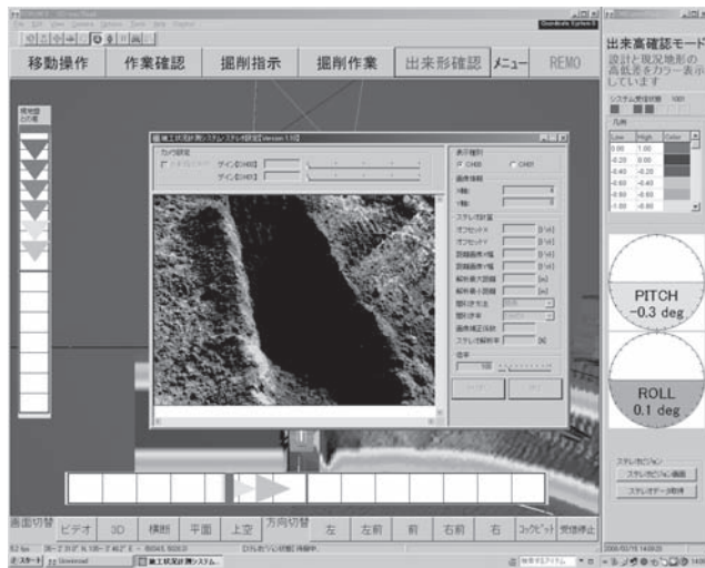
図一2 ステレオビジョンによる計測結果
