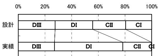
図-1 静岡県の四万十帯における支保構造の変更状況
