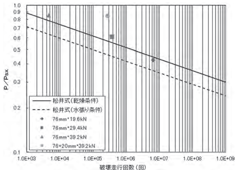
図一 破壊走行回数と荷重比 (P/Psx) の関係
