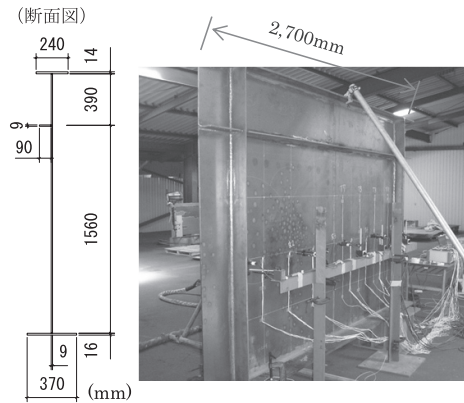
図一6 鋼Iげた模擬試験体
