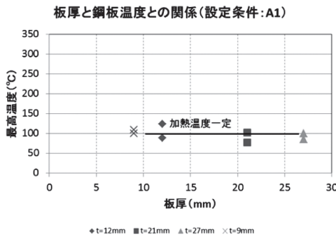
図一4 板厚と鋼板温度の関係
