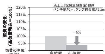
図-12 積み高さの違いと燃費の関係
