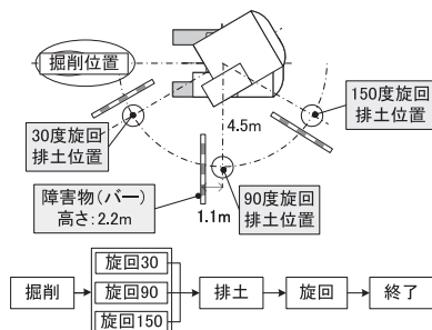
図-7 旋回角度比較試験方法
