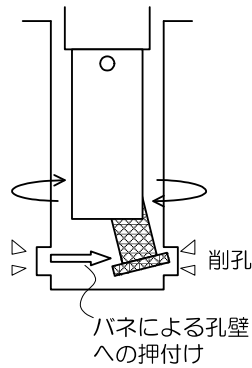
図-2 溝切り方法の模式図
