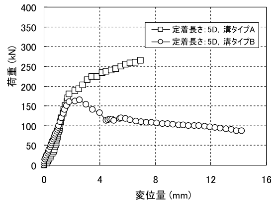
図—6 変位－荷重関係（定着長さ 5D）
