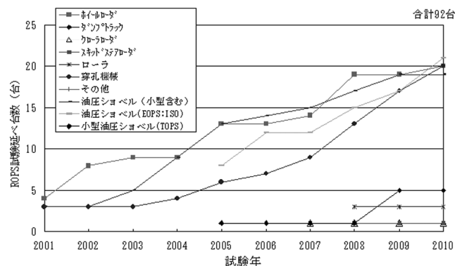
図一 4 ROPS 等の試験実績
