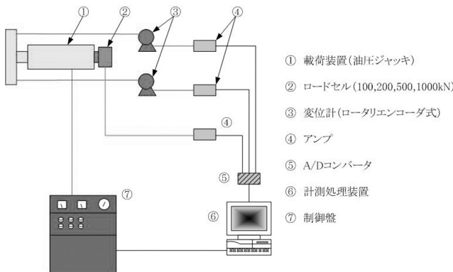
図一 3 ROPS 試験装置の計測・制御
