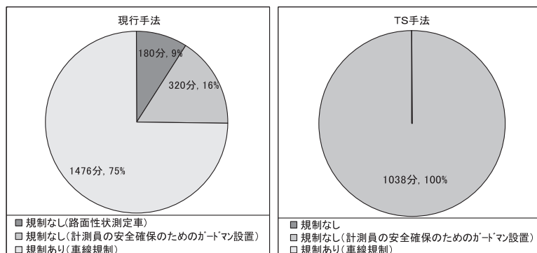
図-4 工事測量に係わる車線規制時間の比較
