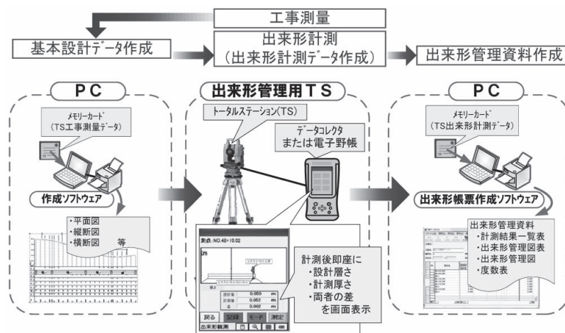
図—1 TSを用いた舗装工の出来形管理の流れ
