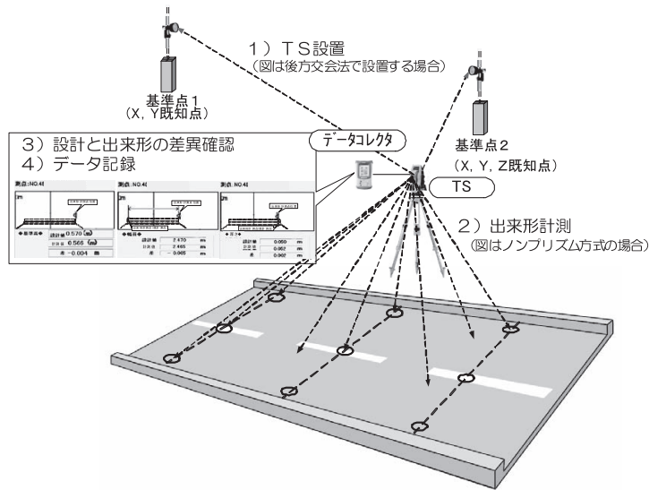
図-2 TSを用いた舗装工の出来形管理手法
